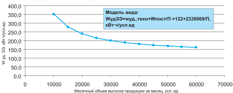
Рисунок 2. Общий вид однофакторной модели удельного электропотребления на выпуск продукции шинного производства
