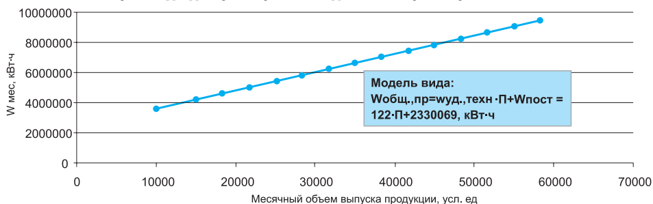
Рисунок 2. Общий вид однофакторной модели удельного электропотребления на выпуск продукции шинного производства
